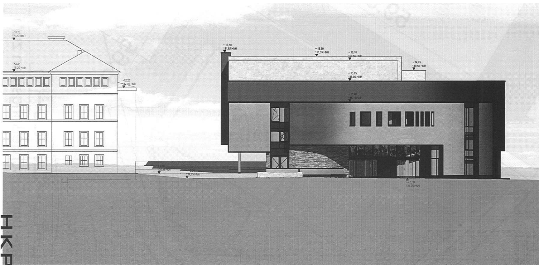
Ansicht Richthofenstraße
