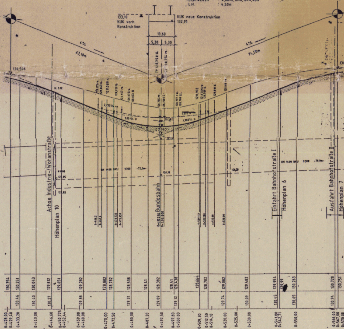
Höhenplan der Eisenbahnbrücke Paulinenstraße
