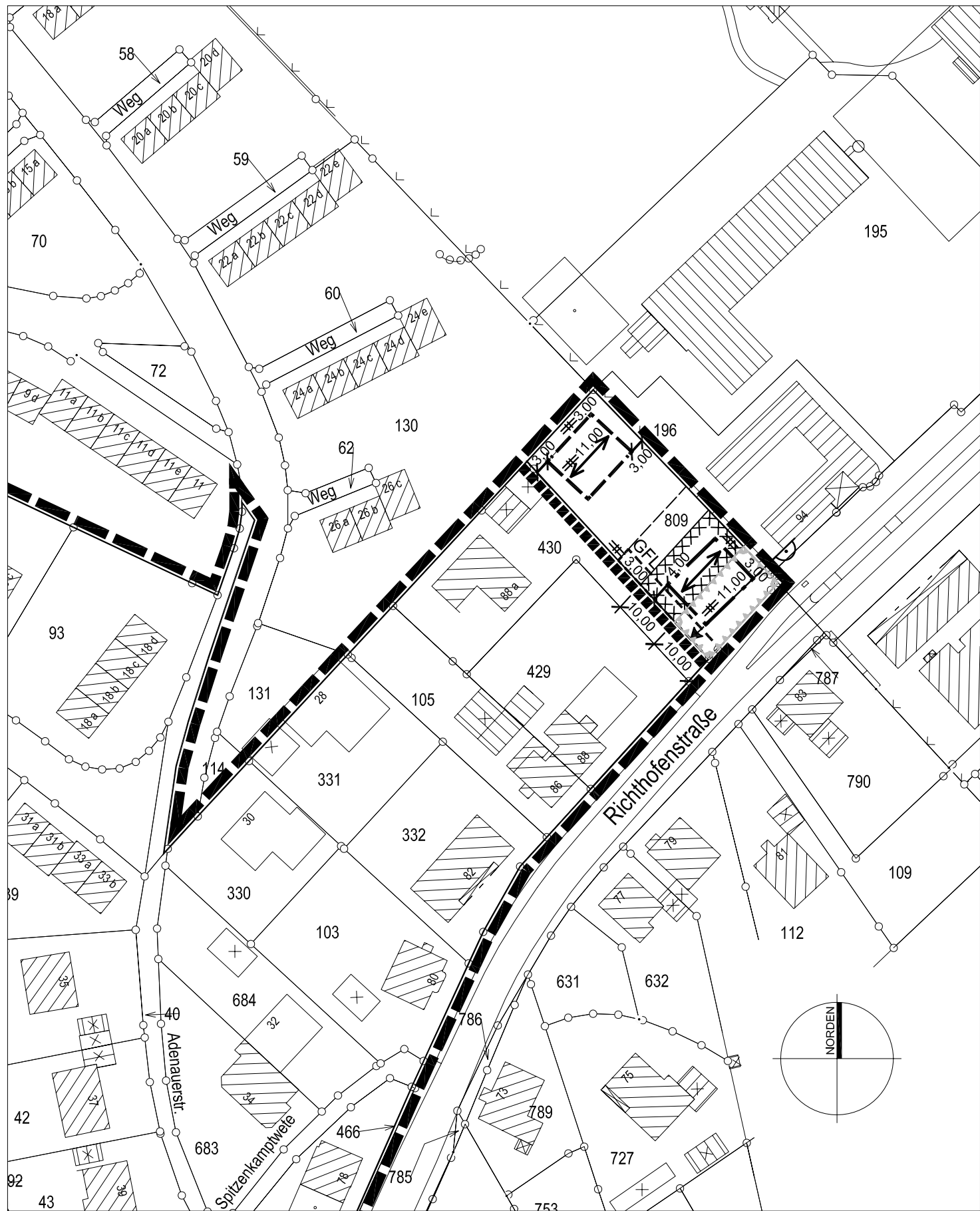
Festlegungsriß
